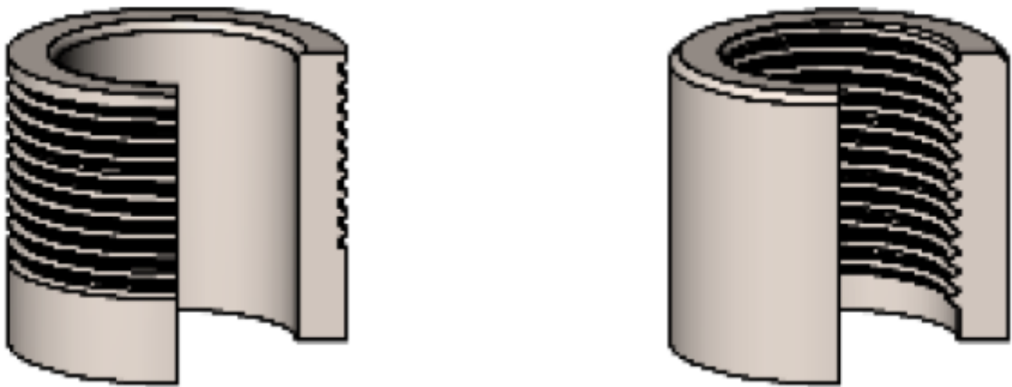
Рис.8 - Резьбовые соединения
